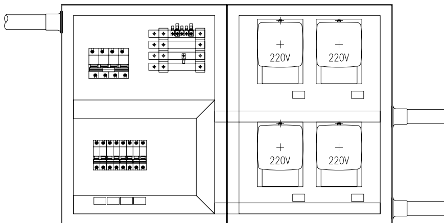
Configuración con 4 Monofásicos
